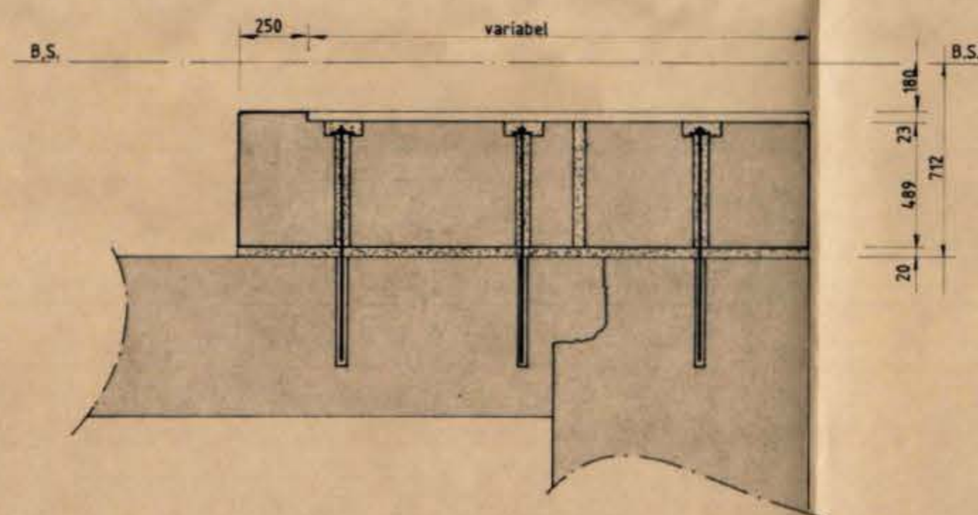
DOORSNEDE A - A
