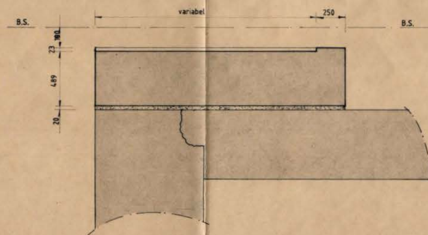
DOORSNEDE B - B
