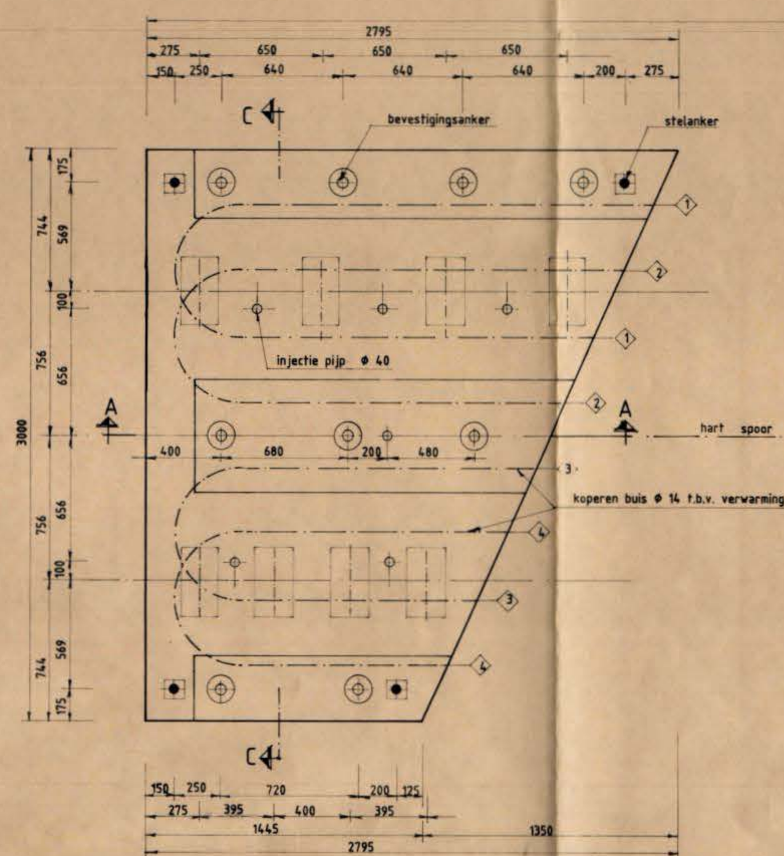
BOVENAANZICHT SPOORPLAATJE TYPE A
