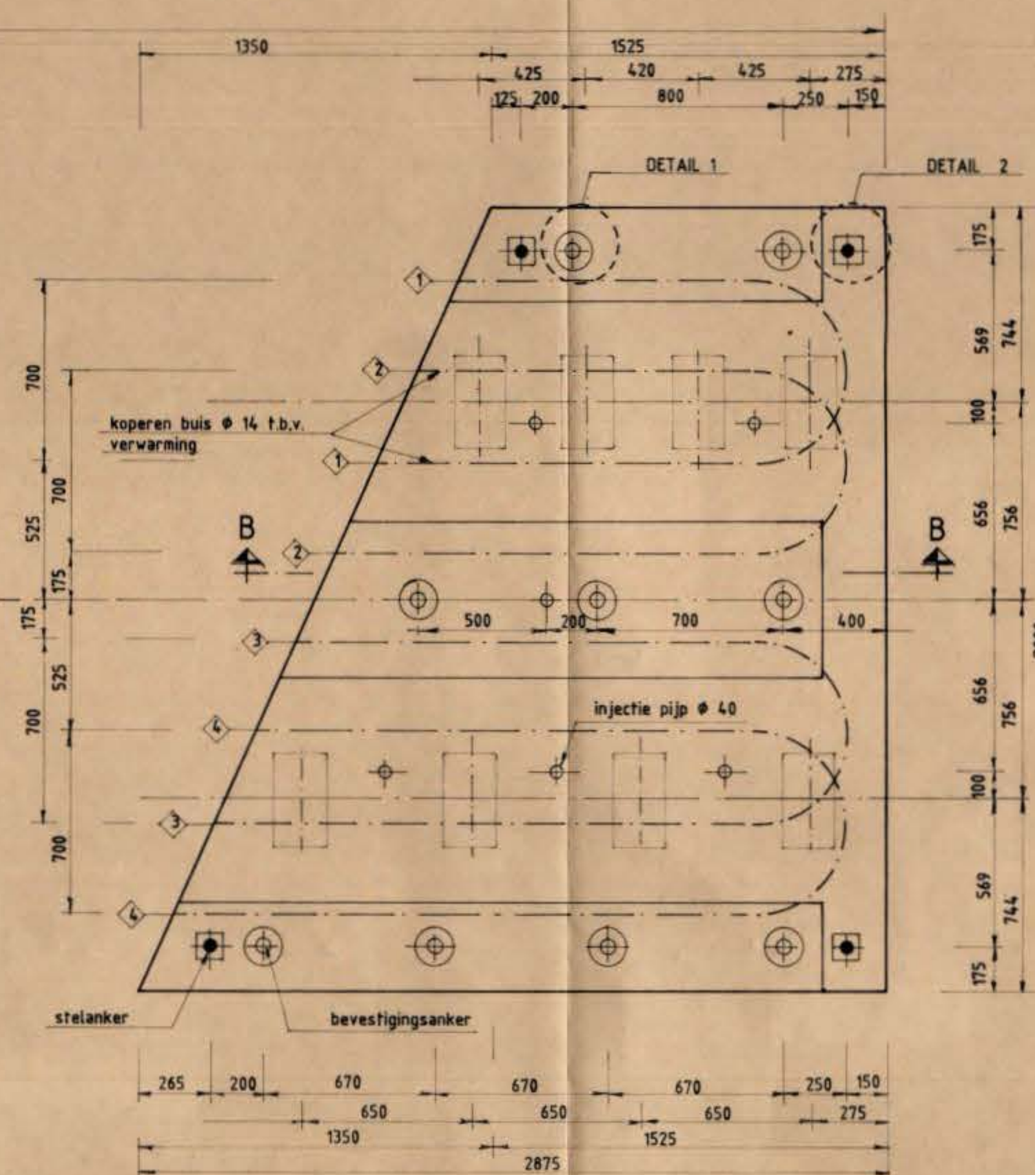
BOVENAANZICHT SPOORPLAATJE TYPE B
